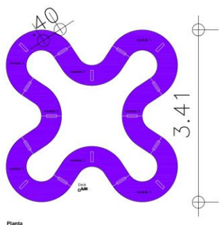
PLANTA DO BANCO PETALA 3 SEM ESCALA
