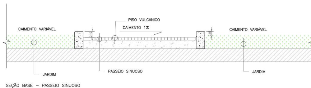
PRAÇA DA CRIANÇA ESC. 1/100
