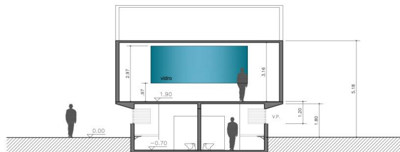
CORTE B 1:100
