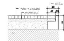
DETALHE PADRÃO DA BORDA ESC. 1/50
