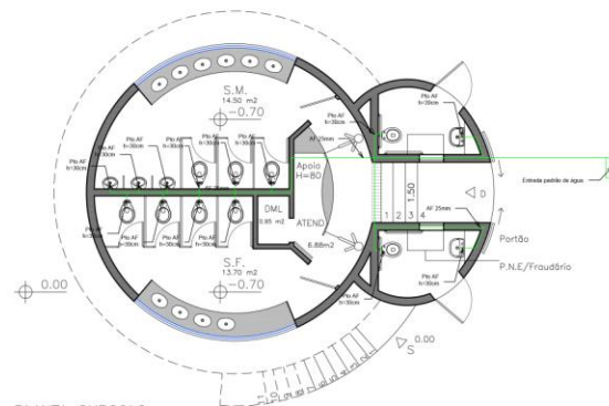
PLANTA SUBSOLO 1:100
