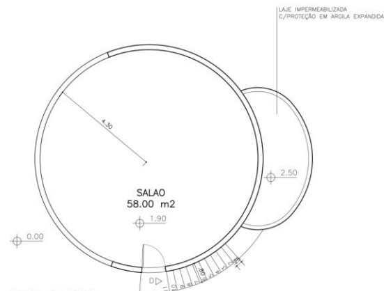
PLANTA SUPERIOR 1:100
