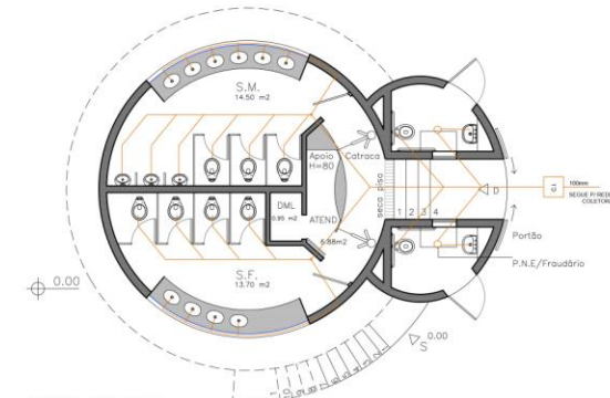
PLANTA SUBSOLO 1:100
