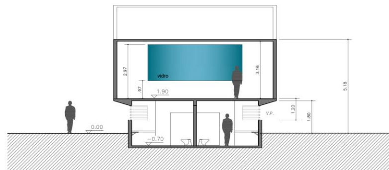
CORTE B 1:100
