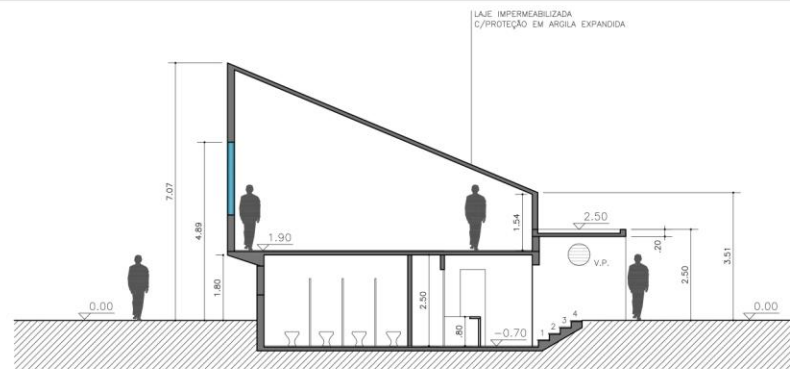
CORTE A 1:100
