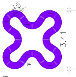
PLANTA DO BANCO PETALA 3 SEM ESCALA
