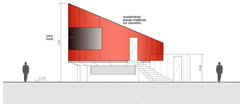
ELEVAÇÃO 1 1:100
