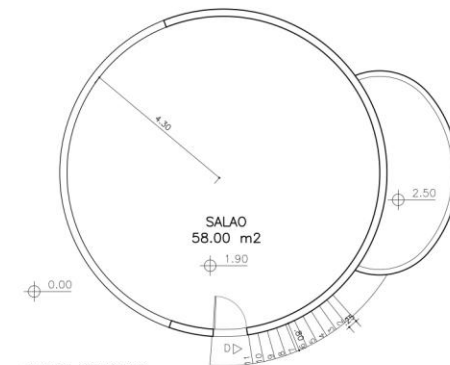
PLANTA SUPERIOR 1:100
