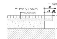
DETALHE PADRÃO DA BORDA ESC. 1/50
