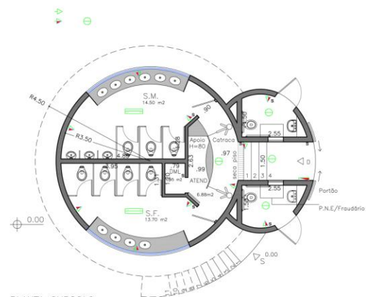
PLANTA SUBSOLO 1:100
