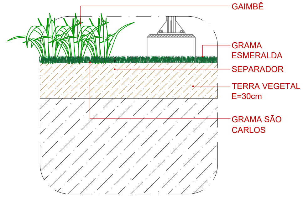
DETALHE 6 Escala 1/20
