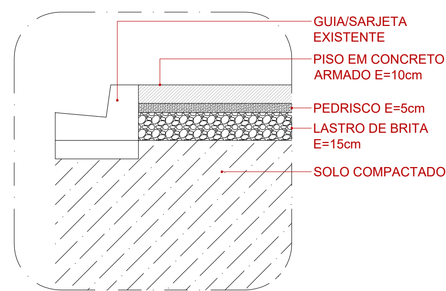
DETALHE 1 Escala 1/20
