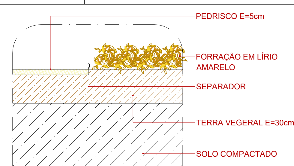
DETALHE 4 Escala 1/20
