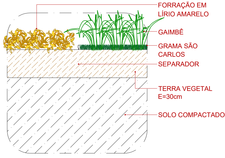
DETALHE 5 Escala 1/20
