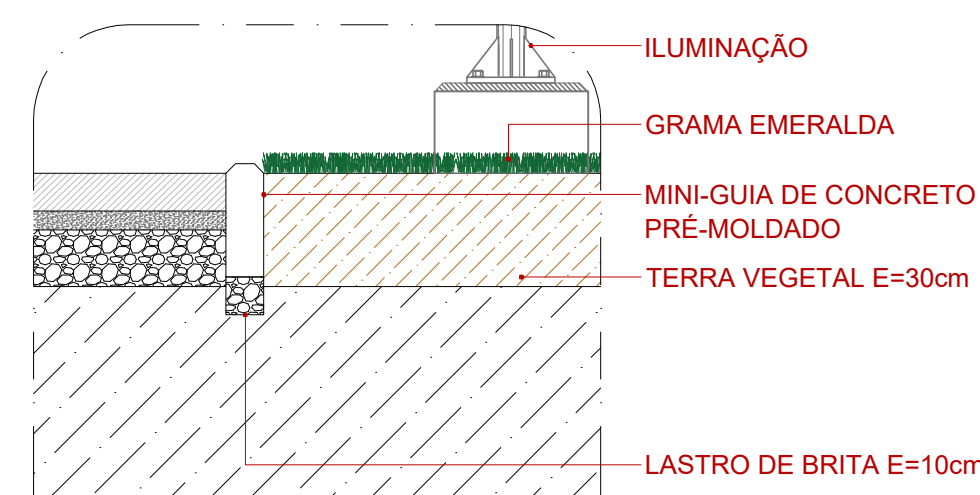
DETALHE 2 Escala 1/20
