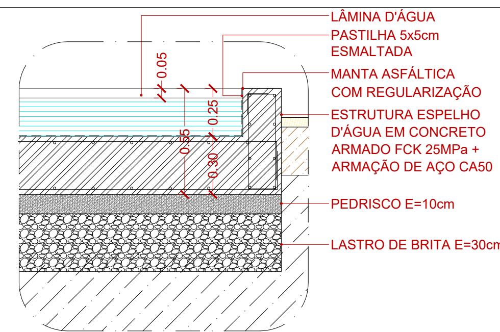
DETALHE 3 Escala 1/20
