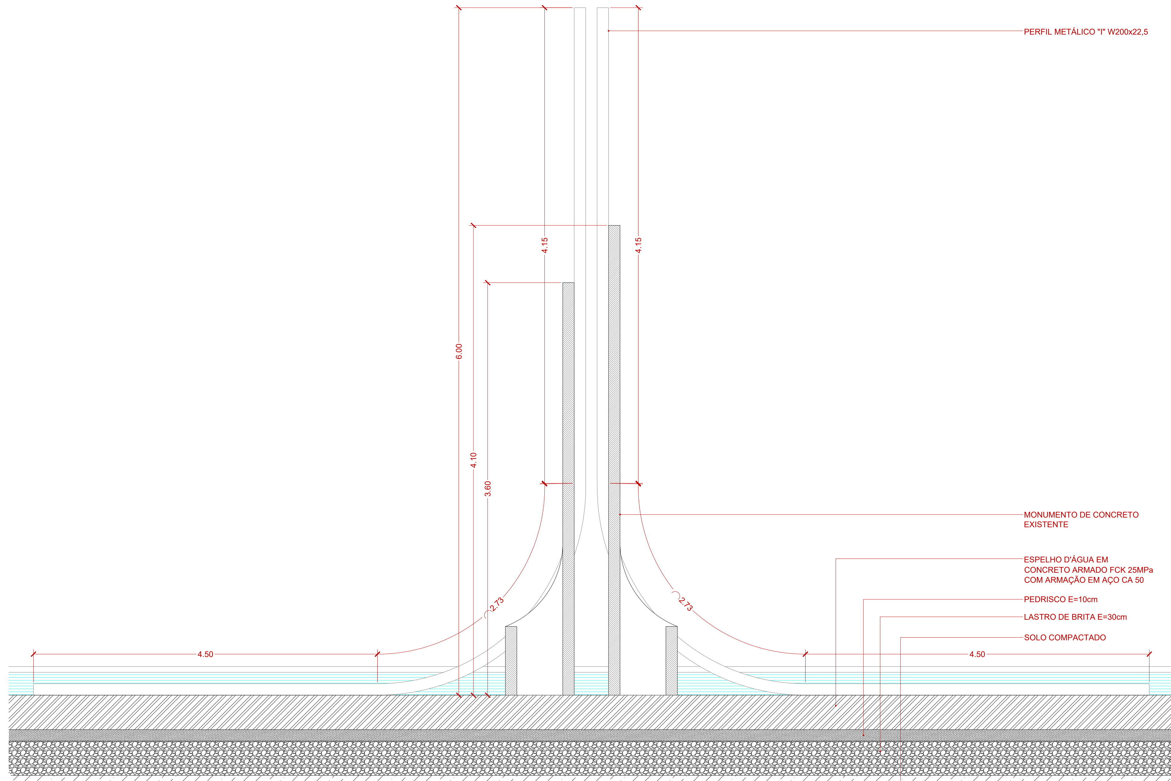
DETALHE 7 Escala 1/20
