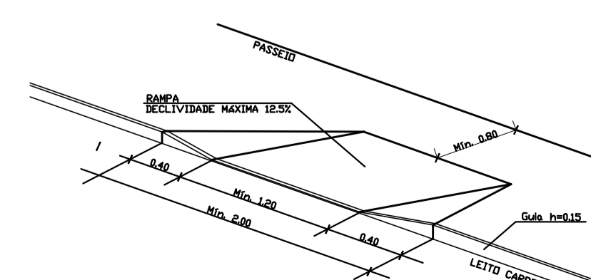
ACESSIBILIDADE NBR 9050 - PERSPECTIVA DA GUIA REBAIXADA SEM ESCALA
