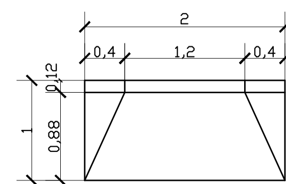
PLANTA DA GUIA REBAIXADA SEM ESCALA
