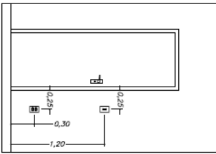
DETALHE GÊNICO DE POSICIONAMENTO DE PONTOS SANE
