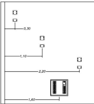
DETALHE GÊNICO DE POSICIONAMENTO DE PONTOS SANE
