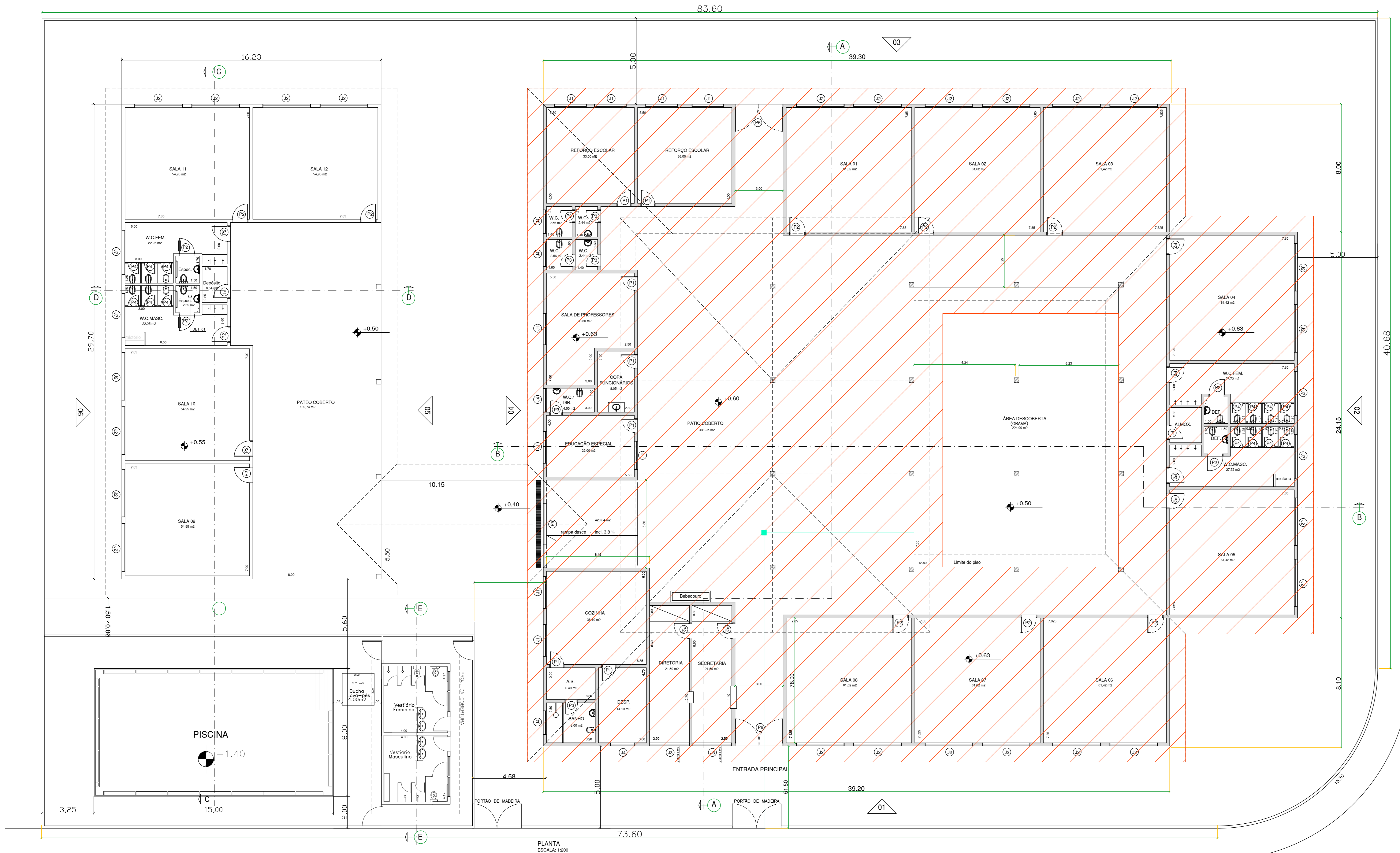
PLANTA ESCALA: 1:200
