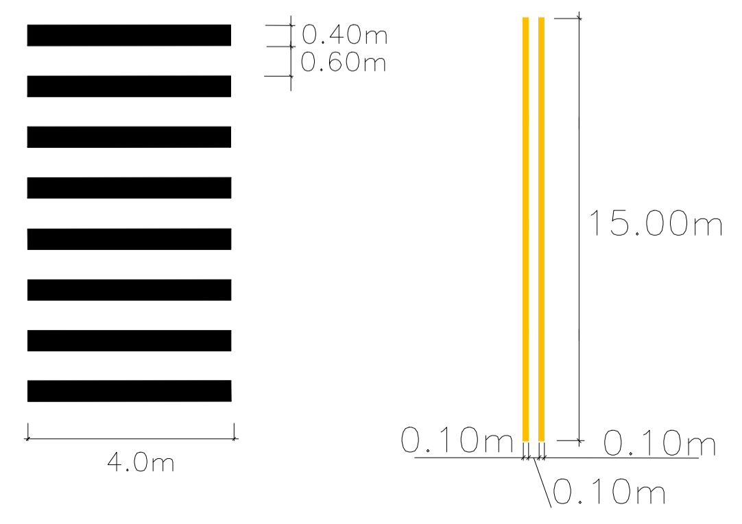
DETALHE DE SINALIZAÇÃO HORIZONTAL DETALHE A DETALHE B
