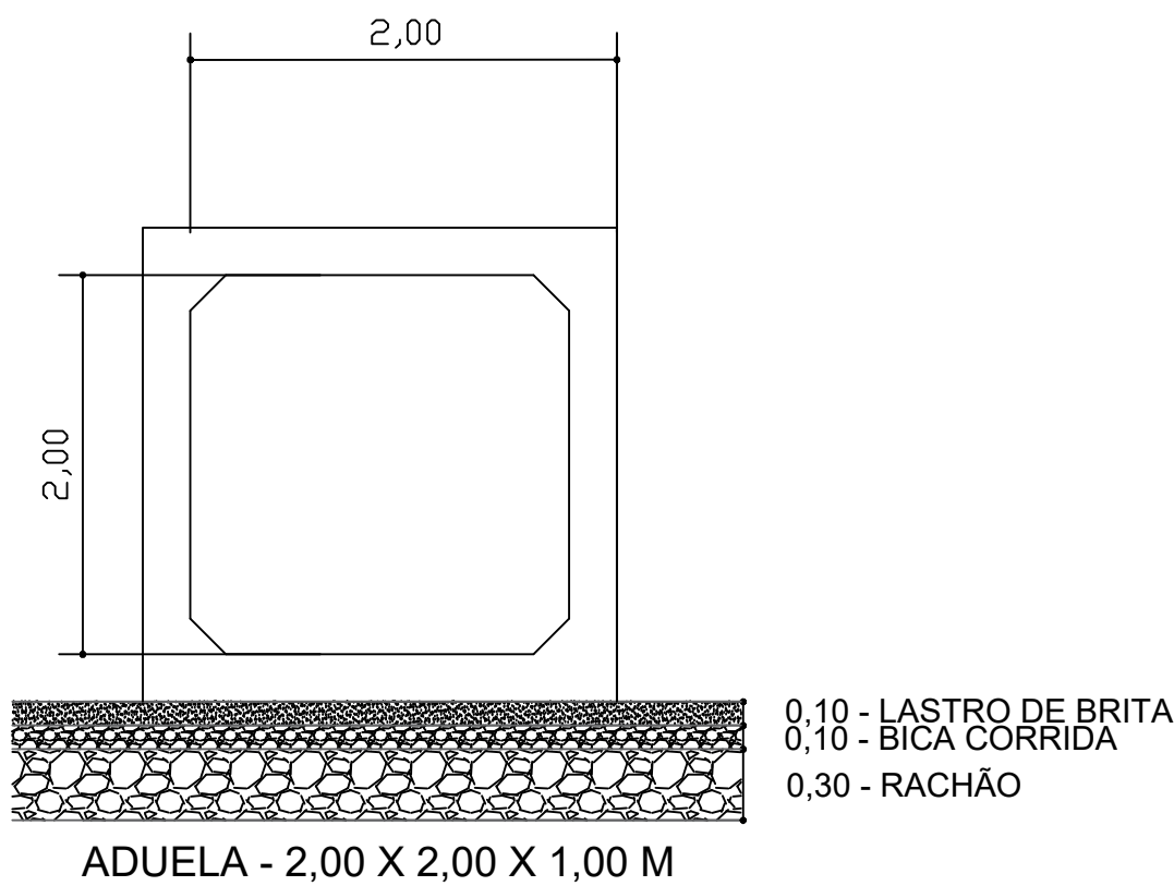
ADUELA - 2,00 X 2,00 X 1,00 M
