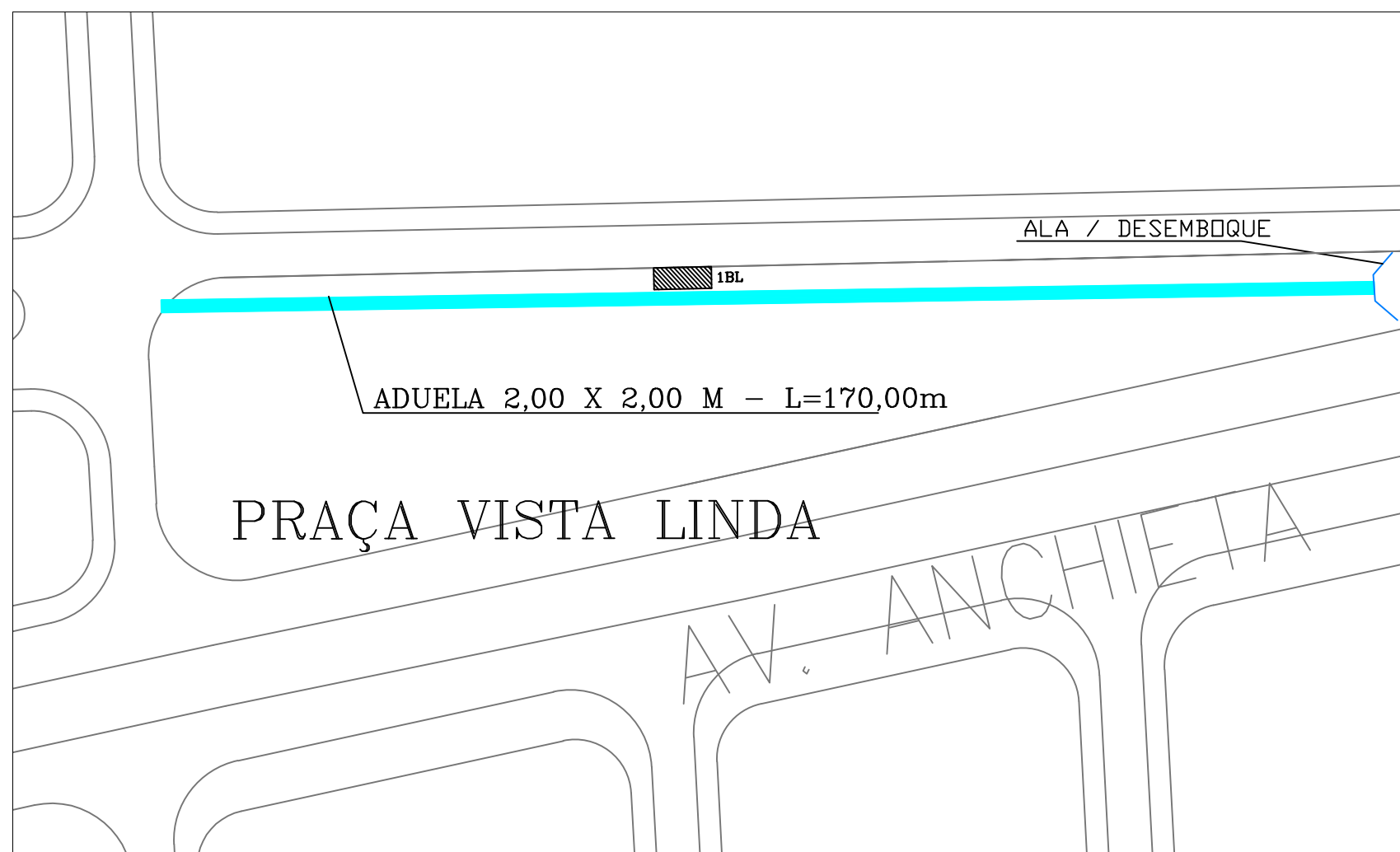
ADUELA - 2,00 X 2,00 X 1,00 M
