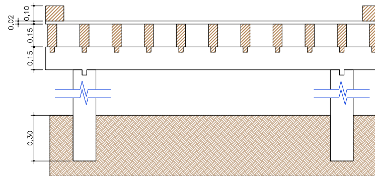
CORTE TÍPICO JJ DETALHE TIPO PASSARELAS PARQUE ESC 1/25
