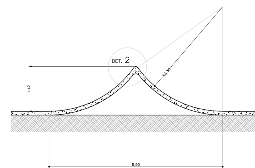
CORTE C - OBSTÁCULO 2 ESC.: 1:50
