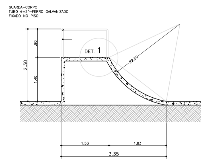
CORTE - OBSTÁCULO 1 ESC.: 1:50
