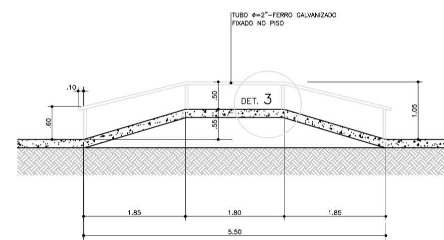
CORTE A - OBSTÁCULO 2 ESC.: 1:50
