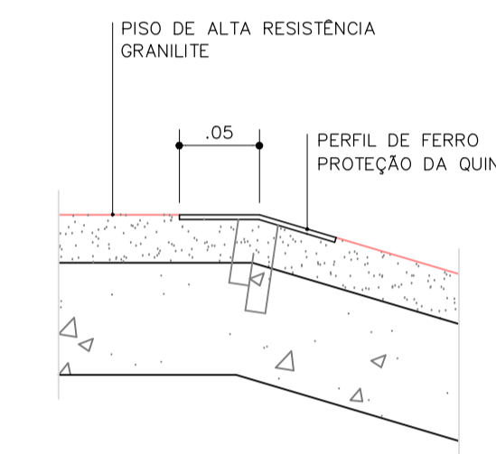
DETALHE 3 CORTE ESQUMÁTICO ESC.: 1:5
