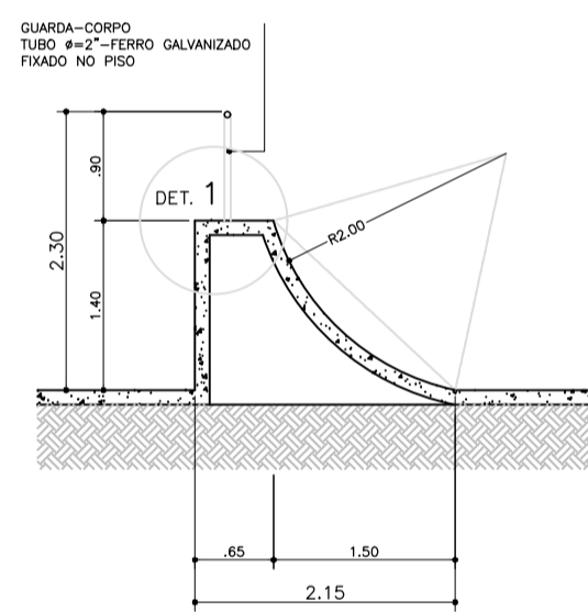
CORTE - OBSTÁCULO 3 ESC.: 1:50
