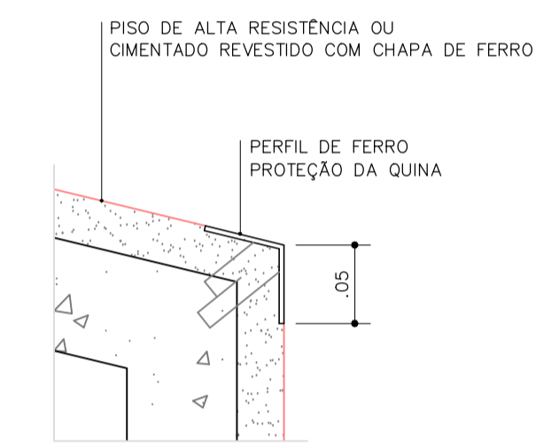
DETALHE 4 CORTE ESQUMÁTICO ESC.: 1:5
