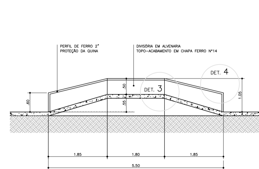
CORTE B - OBSTÁCULO 2 ESC.: 1:50
