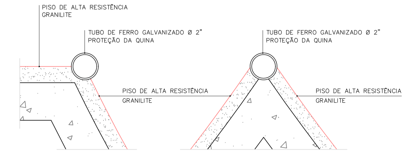
DETALHE 1 CORTE ESQUMÁTICO ESC.: 1:5
