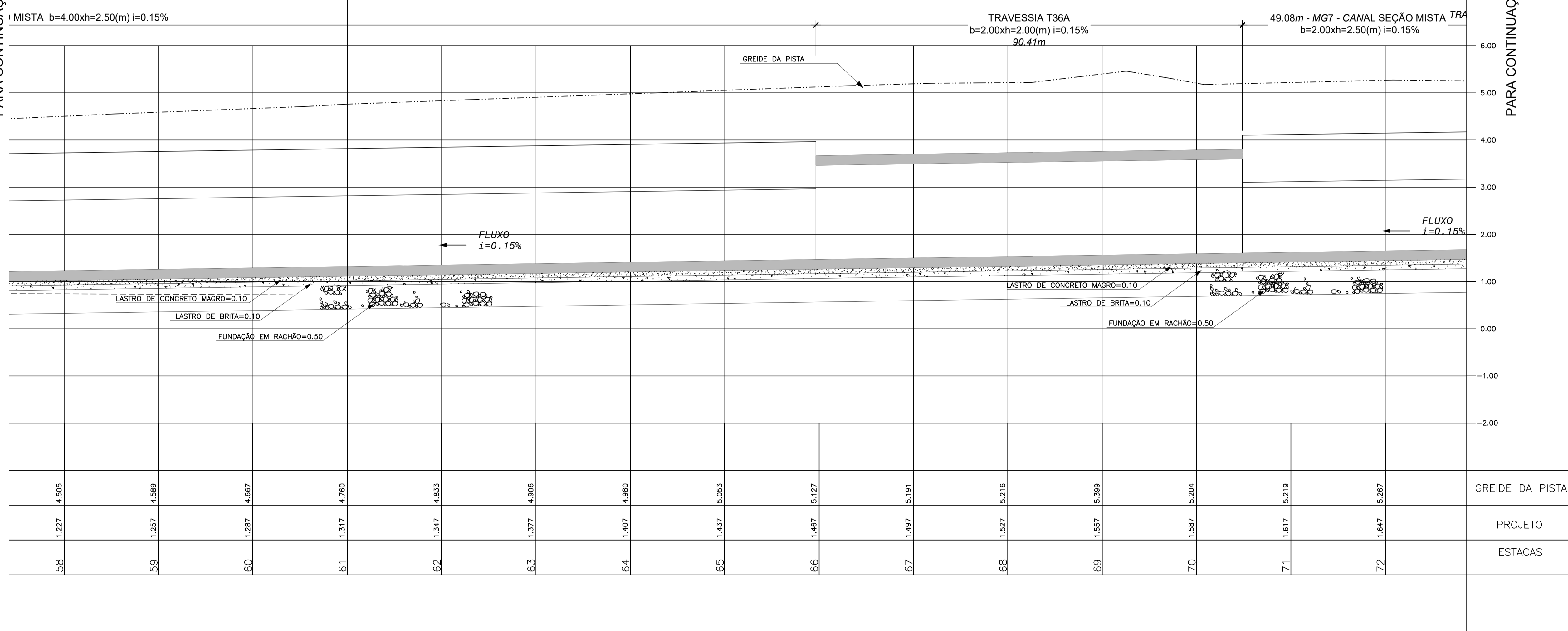
PERFIL LONGITUDINAL ESC.: H=1:500 V=1:50
