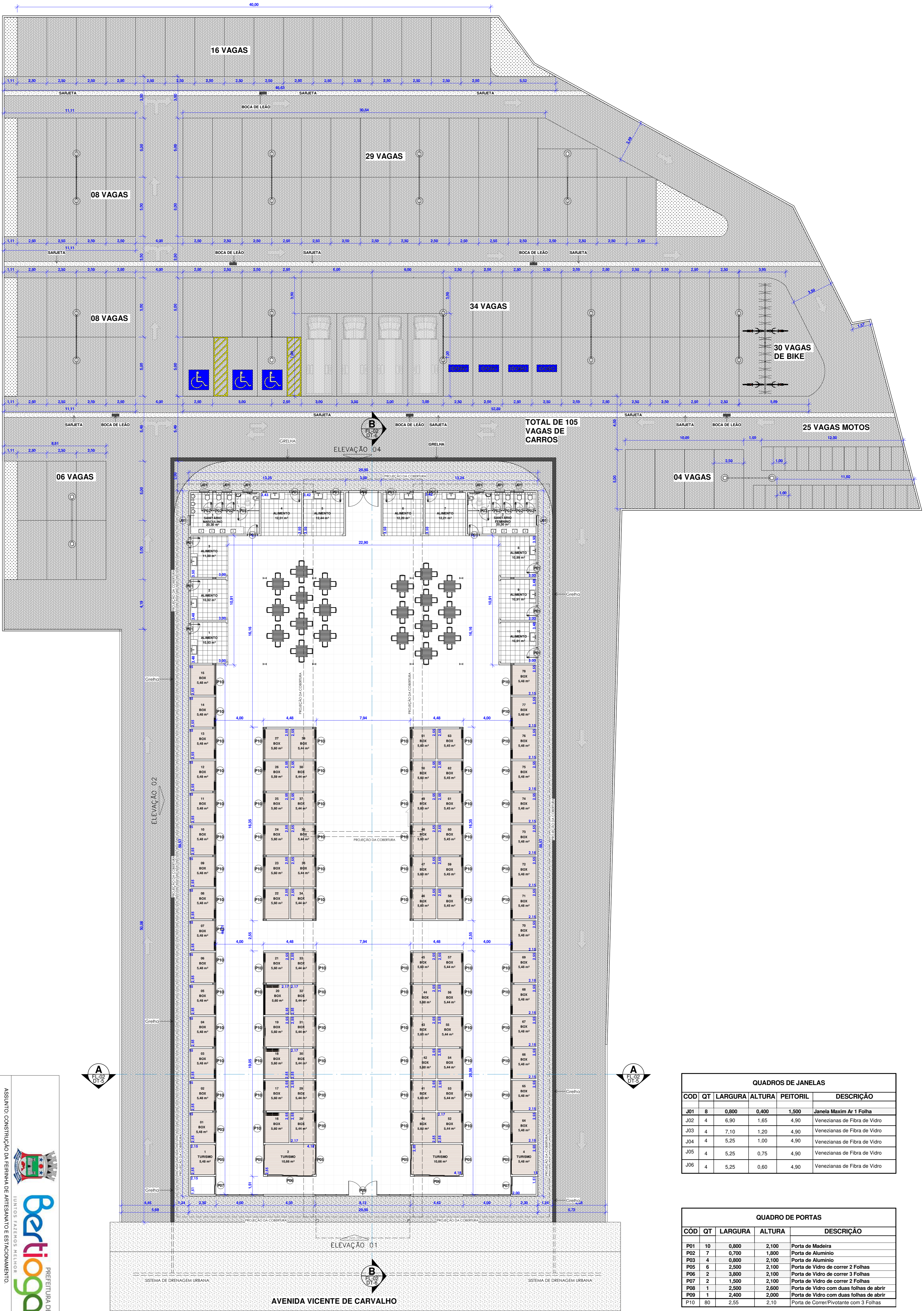
1 TÉRREO ESCALA 1:150
