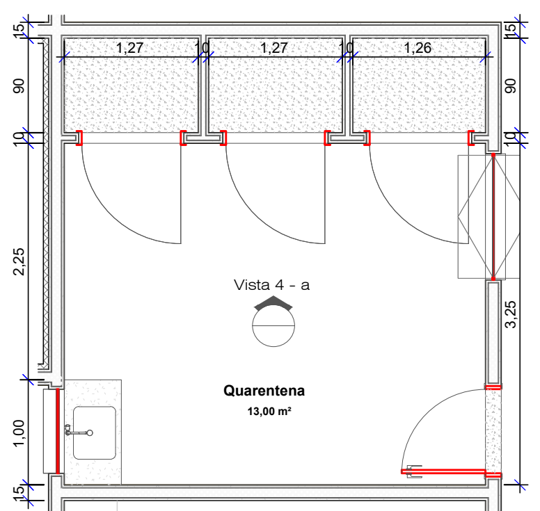
2 PLANTA BAIXA - CHAMADA DE DETALHE 2 ESCALA 1:50
