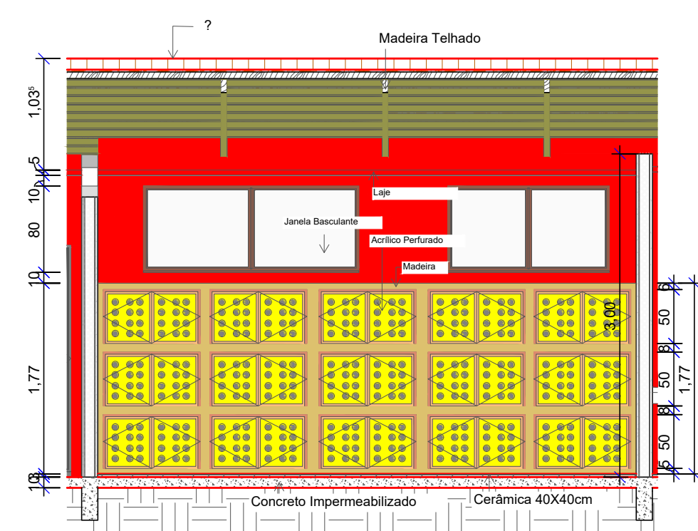
1 VISTA 1 ESCALA 1:50
