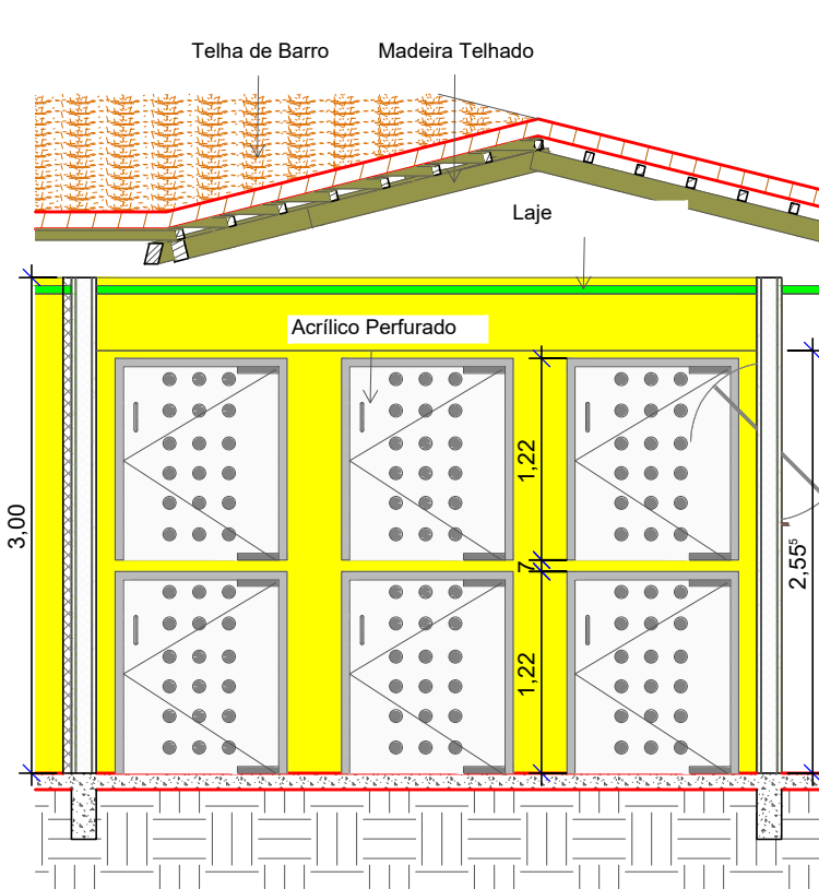
2 PLANTA BAIXA - CHAMADA DE DETALHE 1 ESCALA 1:50
