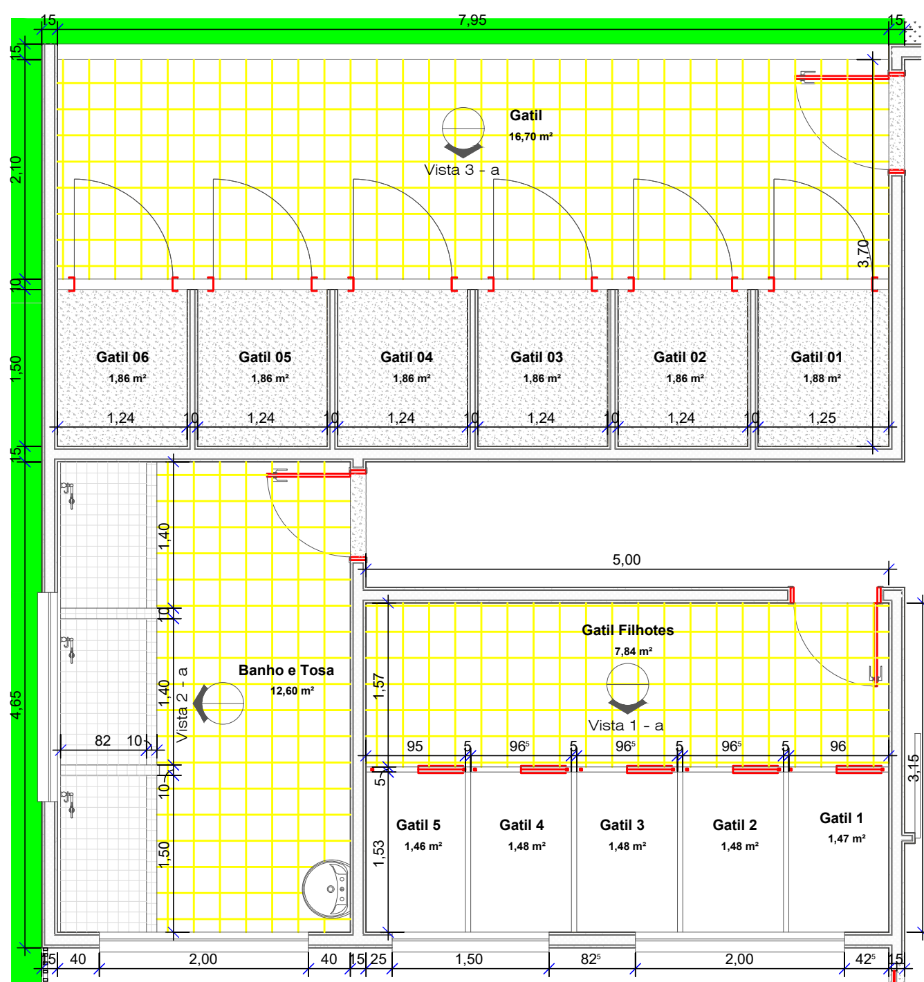
2 PLANTA BAIXA - CHAMADA DE DETALHE 1 ESCALA 1:50
