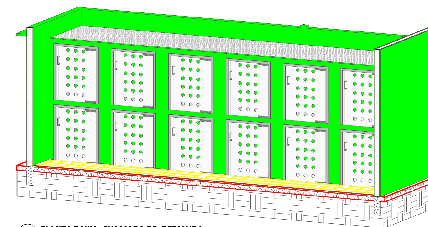
2 PLANTA BAIXA - CHAMADA DE DETALHE 1 ESCALA 1:50
