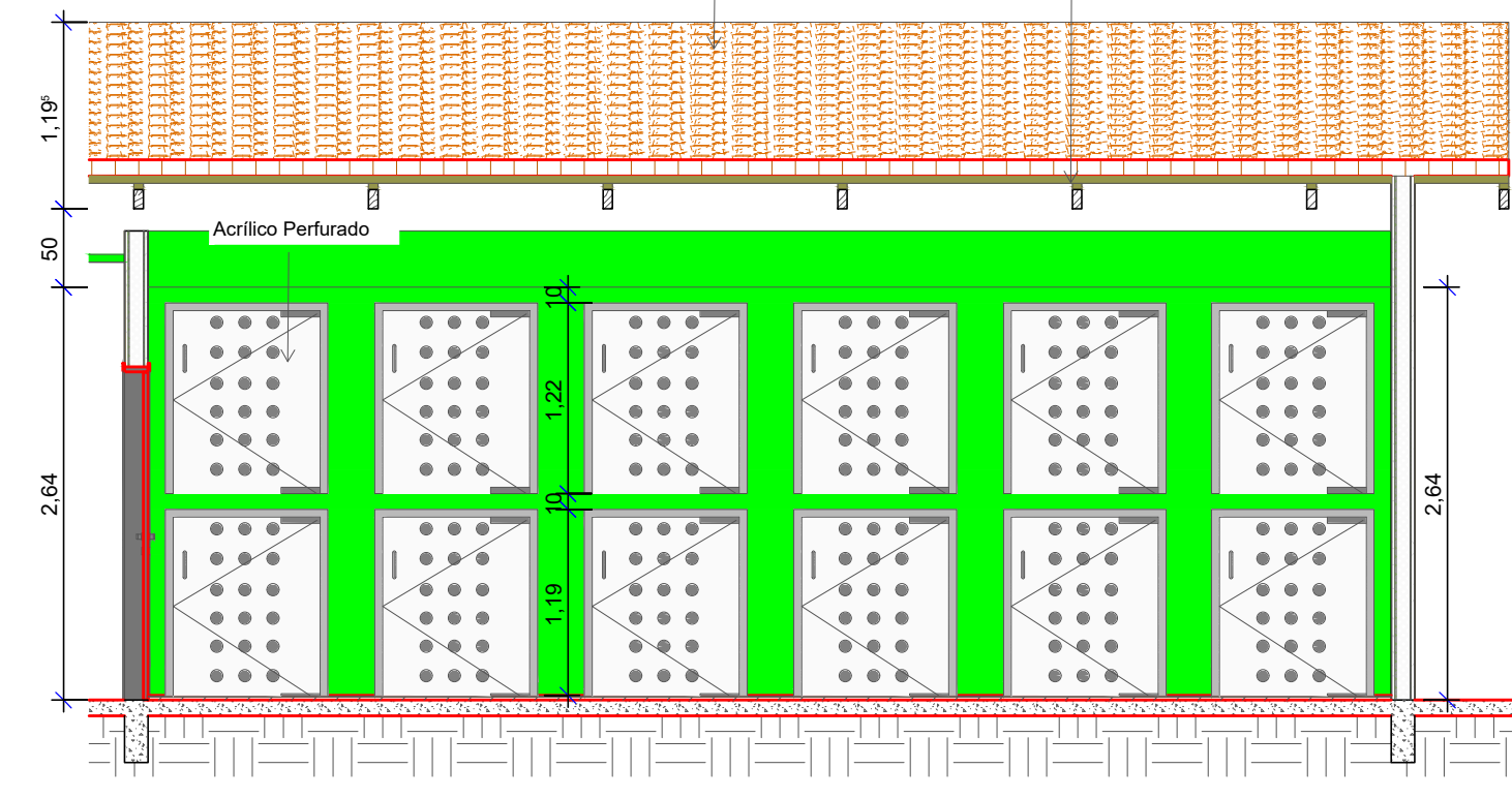
2 PLANTA BAIXA - CHAMADA DE DETALHE 1 ESCALA 1:50
