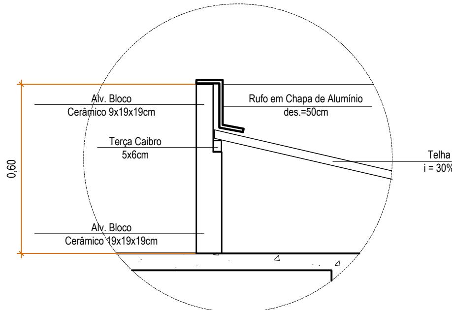
DETALHE 01 (Beiral e Platibanda) SEM ESCALA
