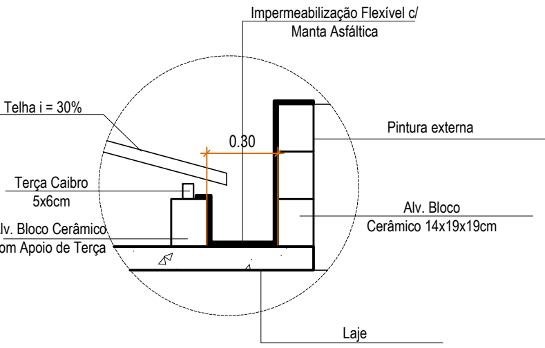
DETALHE 02 (Beiral e Platibanda) SEM ESCALA
