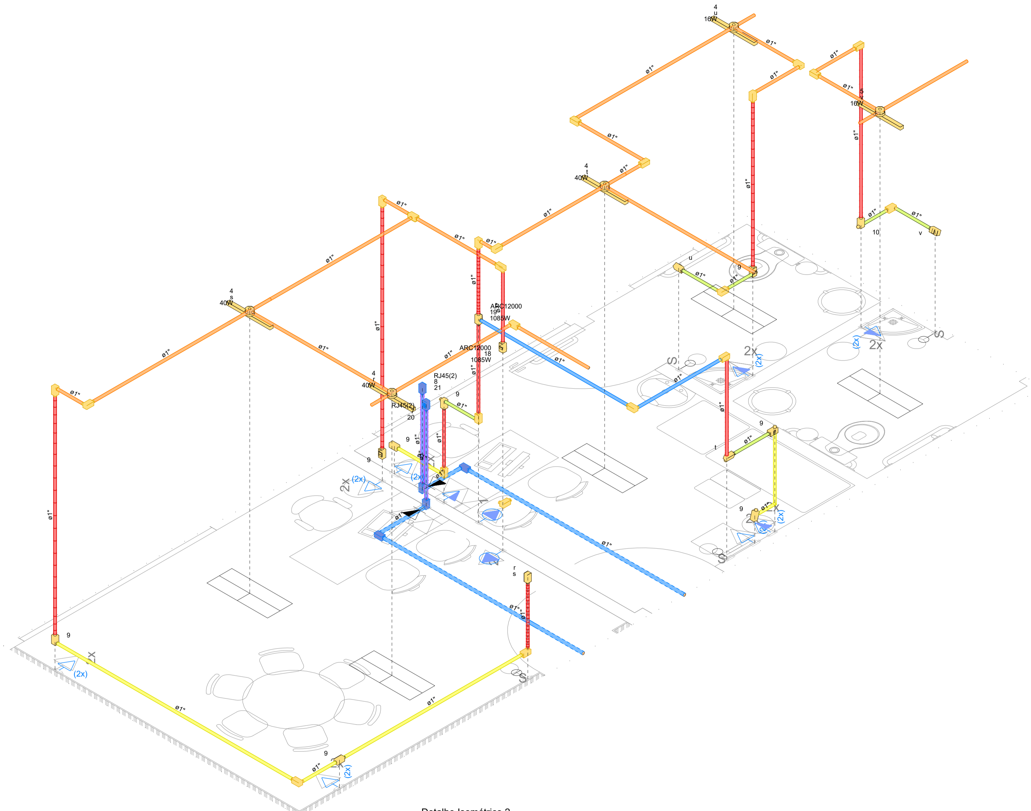
Detalhe Isométrico 2 Escala 1:25
