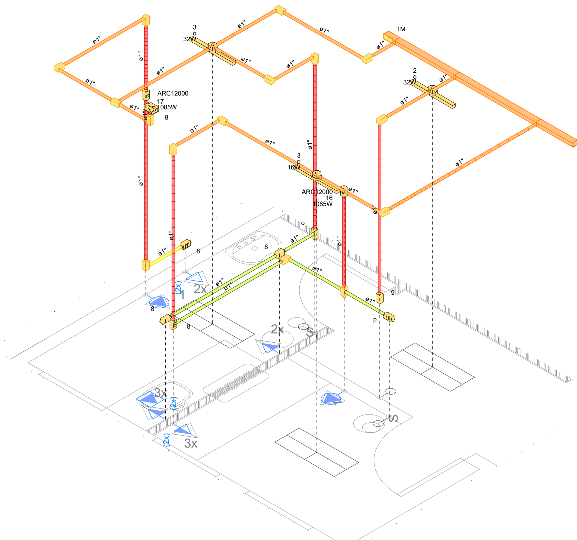
Detalhe Isométrico 1 Escala 1:25
