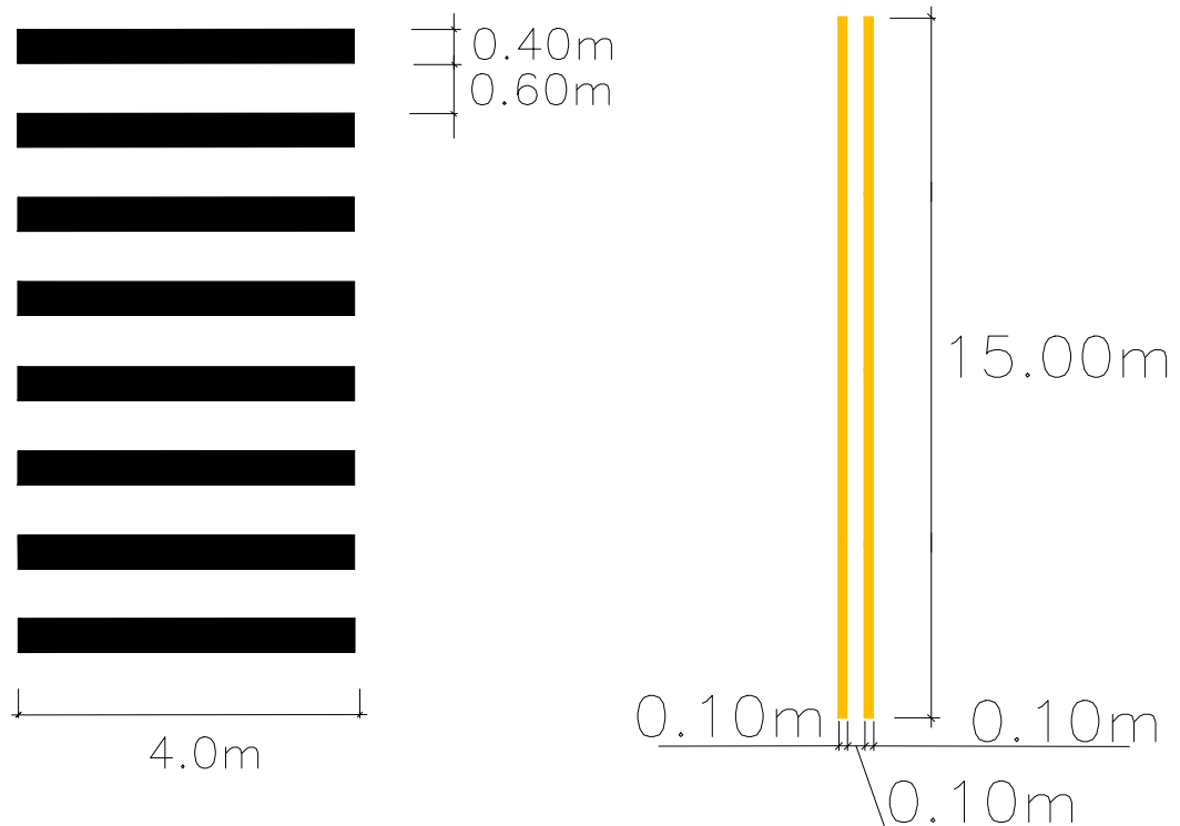
DETALHE DE SINALIZAÇÃO HORIZONTAL
